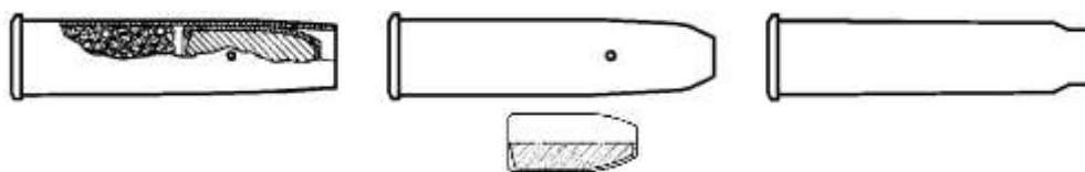
Рис. 1. 7,62-мм патрон к револьверу Наган обр. 1895 г.
