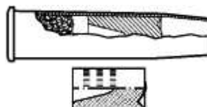
Рис. 2. 7,62-мм спортивный револьверный патрон В-1
